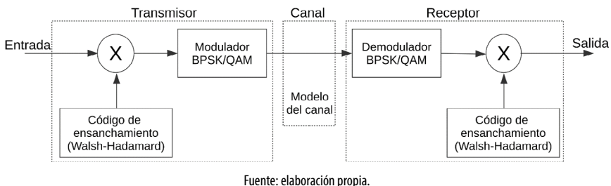
Figura 2. Sistema de comunicaciones usando DSSS
