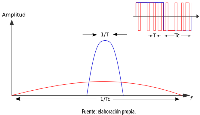
Figura 1. Técnica de modulación DSSS
